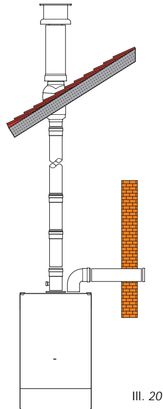
Exemple d'aspiration au mur et évacuation au cheminée
